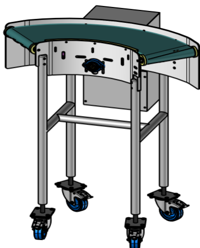
Convoyeur courbe à grille ou à bande
